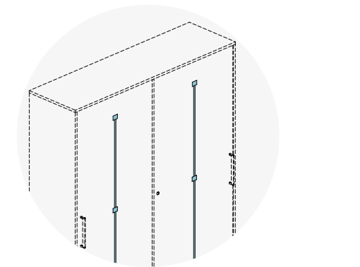
raddrizza ante interno anta h. 160-200 cm inner door strenghtner h.160-200 cm (63" - 78 3/4") barre raidisseuse interne pour porte h. 160-200 cm Innere Türversteifung H.160-200 cm rechtmaker deur binnenkant deur h. 160-200 cm endereza puerta interior h. 160-200 cm.
